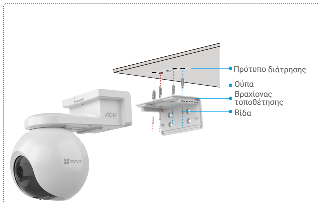
Εικ. 1 Τοποθέτηση στην οροφή
