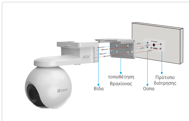
Εικ. 2 Τοποθέτηση στον τοίχο
